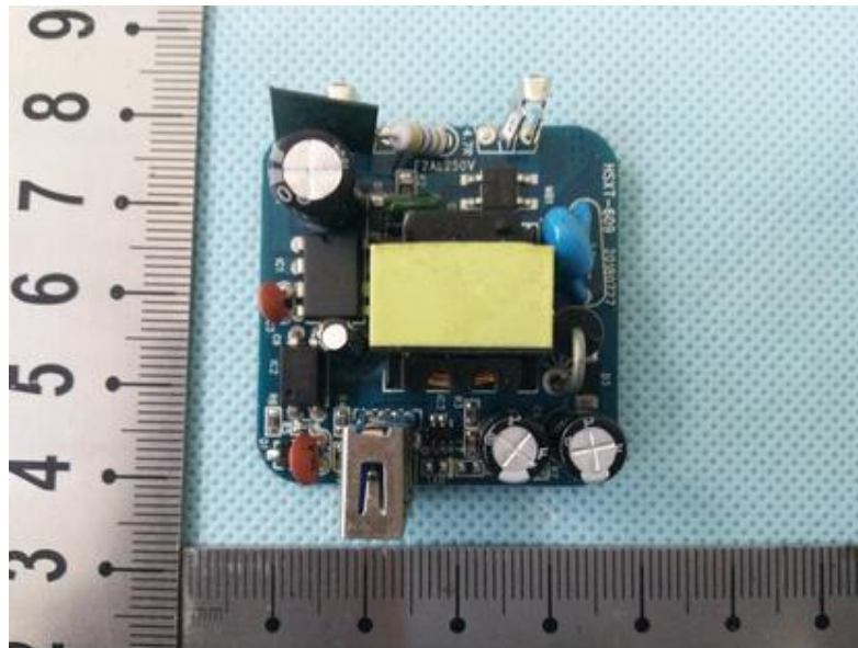
EUT Photo 6
